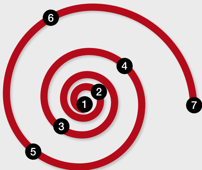
Das Spiralmodell
